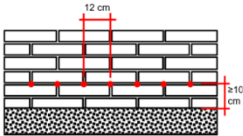
Bohrlochabstände bei gleichmäßigem Mauerwerk im Vergleich bei Sopro Verkieselung Gel (links) und Sopro Verkieselung VK 690 (rechts)
